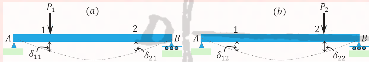
Teorema di reciprocità di Betti per l'elasticità (caso particolare di una trave)
